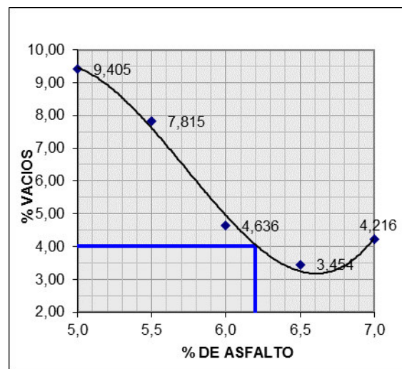
Figura 3. 3 Porcentaje de vacíos en relación al porcentaje óptimo de asfalto
