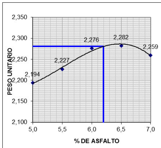
Figura 3. 2 Peso unitario o densidad Bulk en relación al porcentaje óptimo de asfalto
