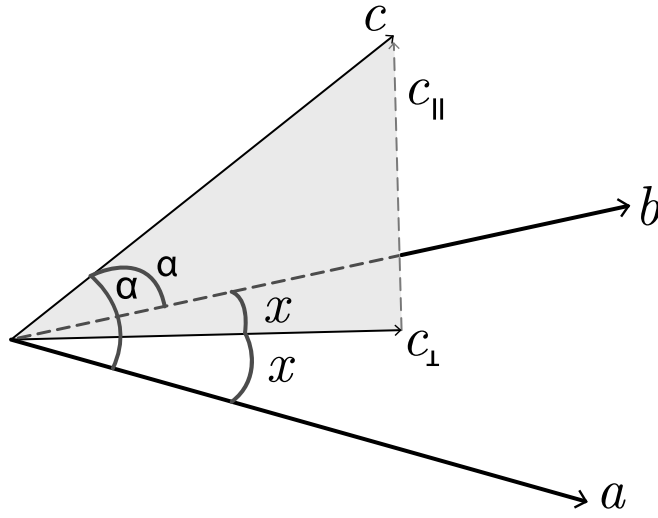
Figura 4.11: Vector bisectriz.
