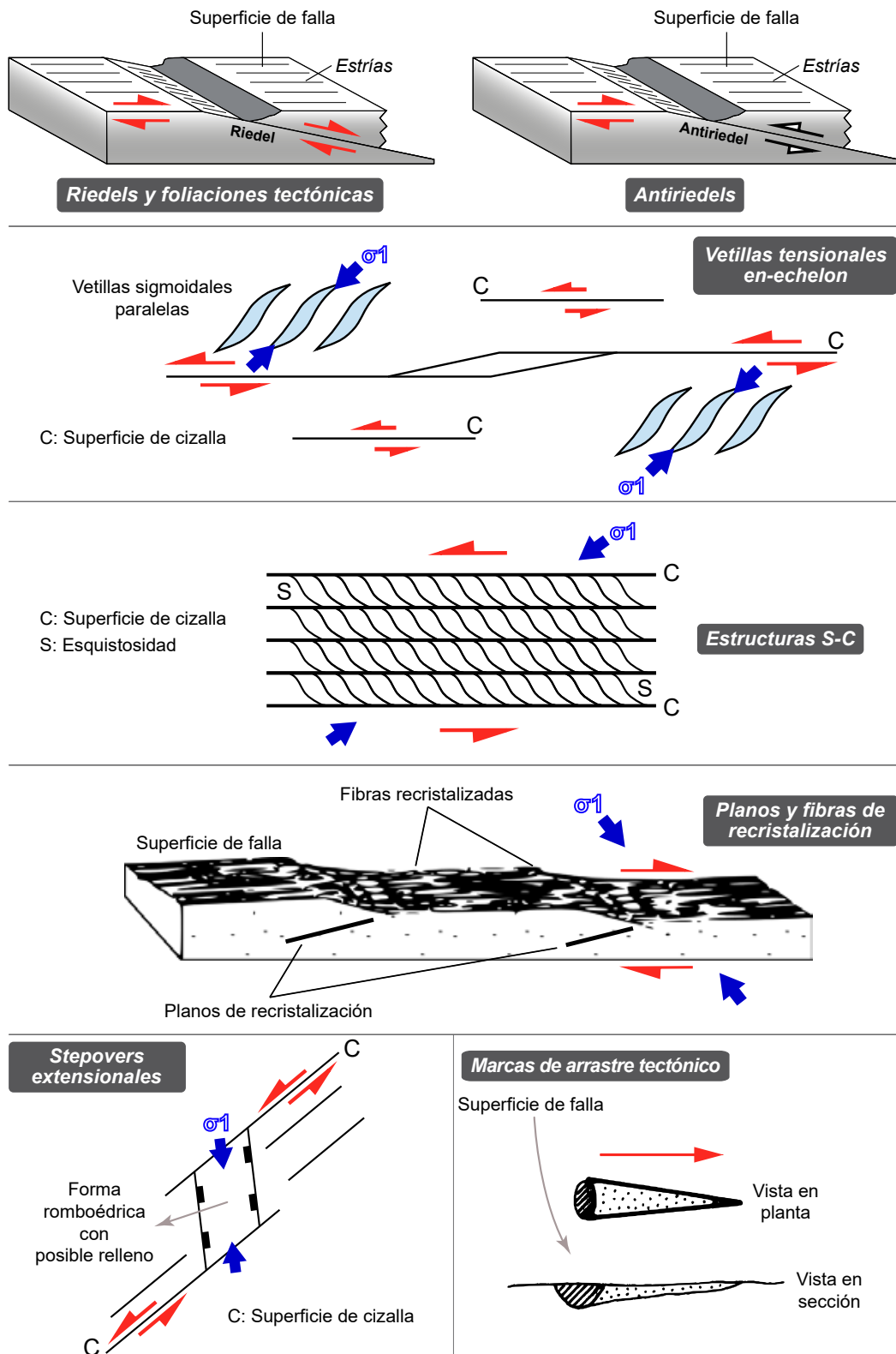
Figura 8. Microlineamientos tectónicos e indicadores cinemáticos. Tomado de Allmendinger (1987), Doblas (1998) y Van Der Pluijm y Marshak (2004).
