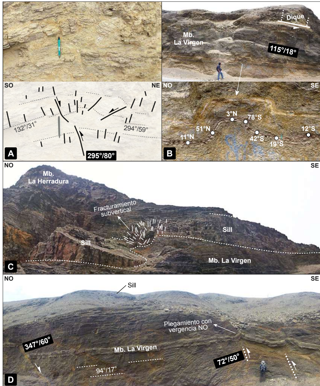
Figura 41. Vistas de campo del mapeo geológico de la Figura 40. A: Anticlinal pequeño en los alrededores de la Falla La Virgen, B: Pliegue “en cofre”, C: Monoclinal en sill que aflora cerca de la Falla Salto del Fraile y D: Alrededores de la Falla La Herradura.
