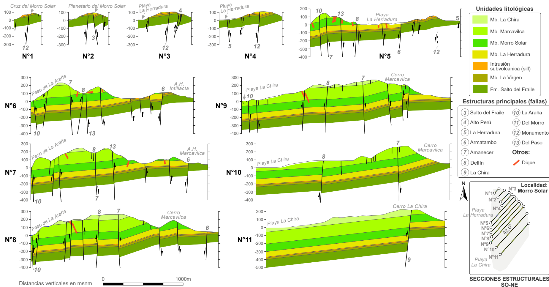
Figura 47. Secciones estructurales SO-NE de azimuth 42.0^\circ en el Morro Solar (ver escala más amplia en el Anexo N°2). Sus longitudes en kilómetros son: N°1=0.34, N°2=0.49, N°3=0.66, N°4=0.79, N°5=1.88, N°6=2.03, N°7=2.22, N°8=2.35, N°9=2.62, N°10=2.40 y N°11=2.22.
