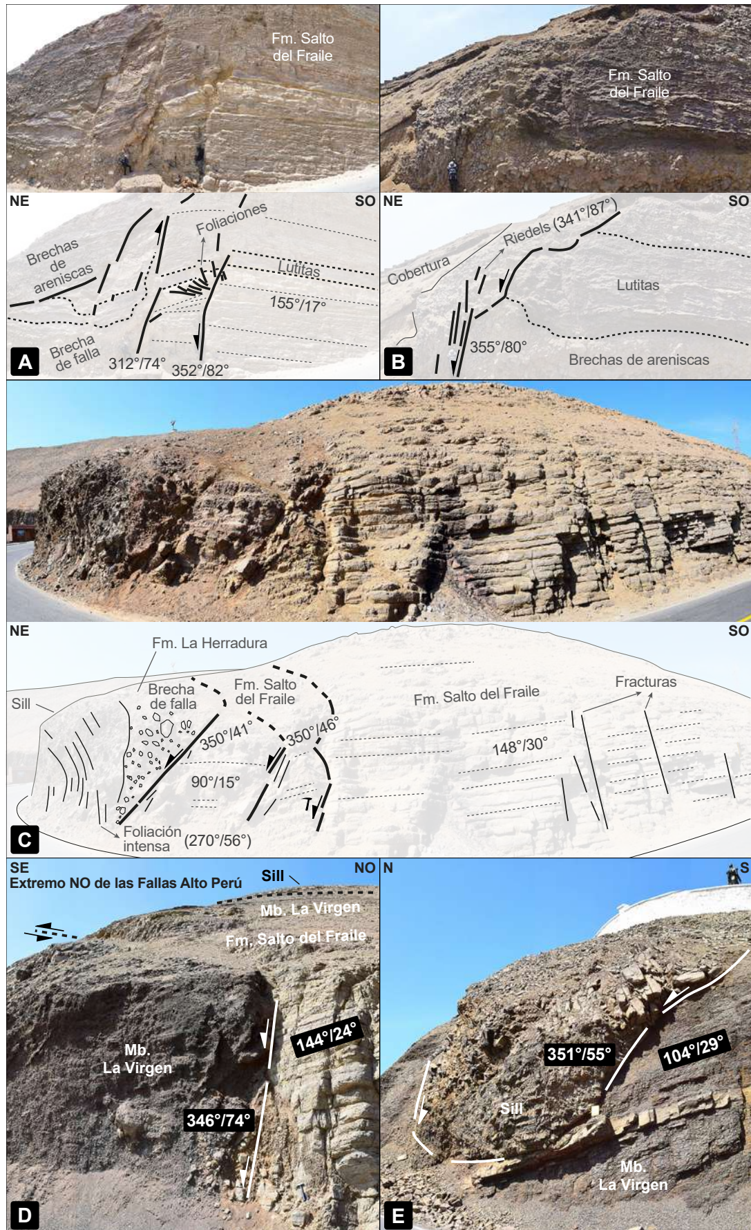
Figura 34. Vistas de campo del mapeo geológico observado en la Figura 32.
