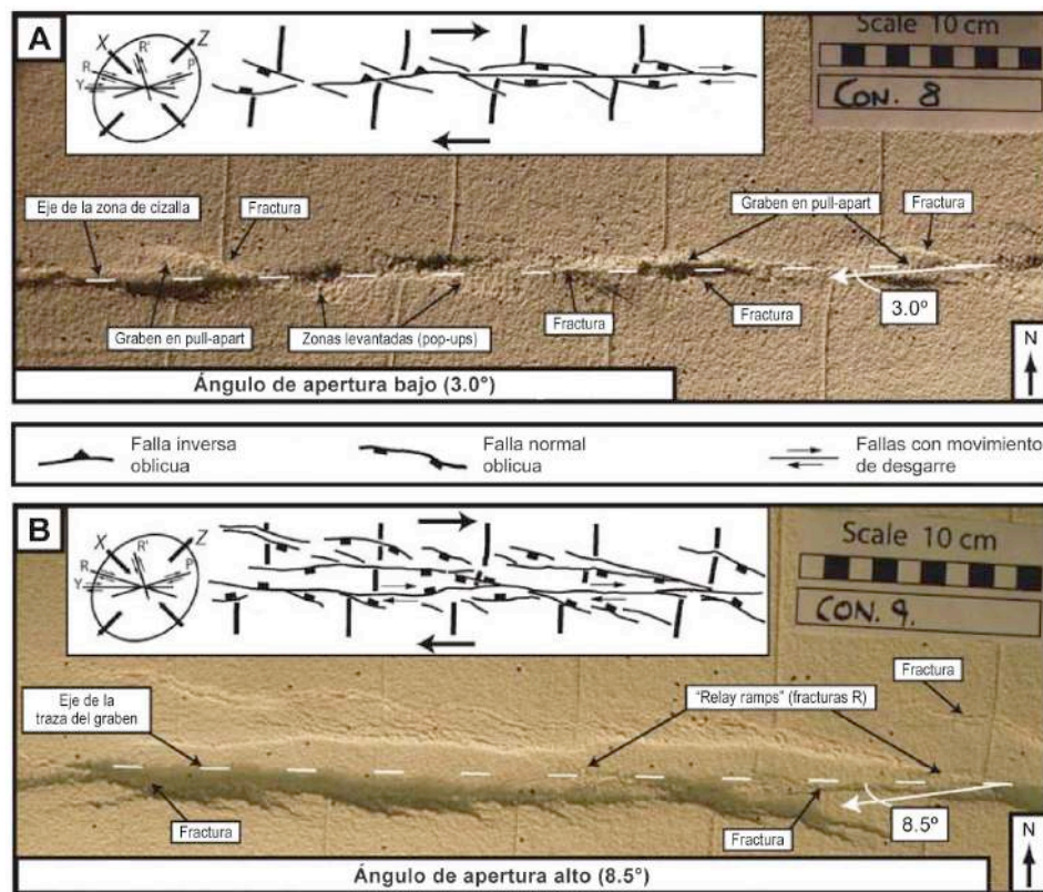
Figura 7. Geometrías de estructuras tectónicas en un modelo analógico. Las estructuras aparecen invariablemente desde un primer orden (escala del modelo) hasta en dimensiones más reducidas (milimétricas). Tomado de Holohan et al. (2008).
