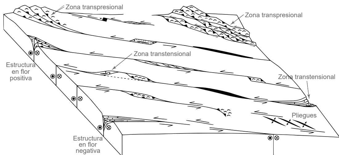
Figura 12. Arquitectura tectónica de fallas de desgarre (Sylvester, 1988) en la que coexisten fallas normales (por transtensión) e inversas (por transpresión). Tomado de Cunningham y Mann (2007).
