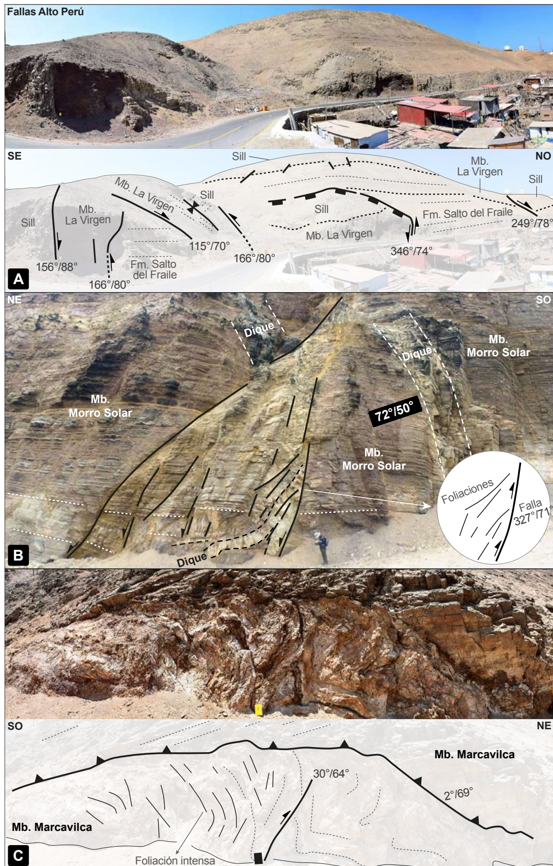
Figura 44. Vistas de campo del mapeo geológico observado en la Figura 43.
