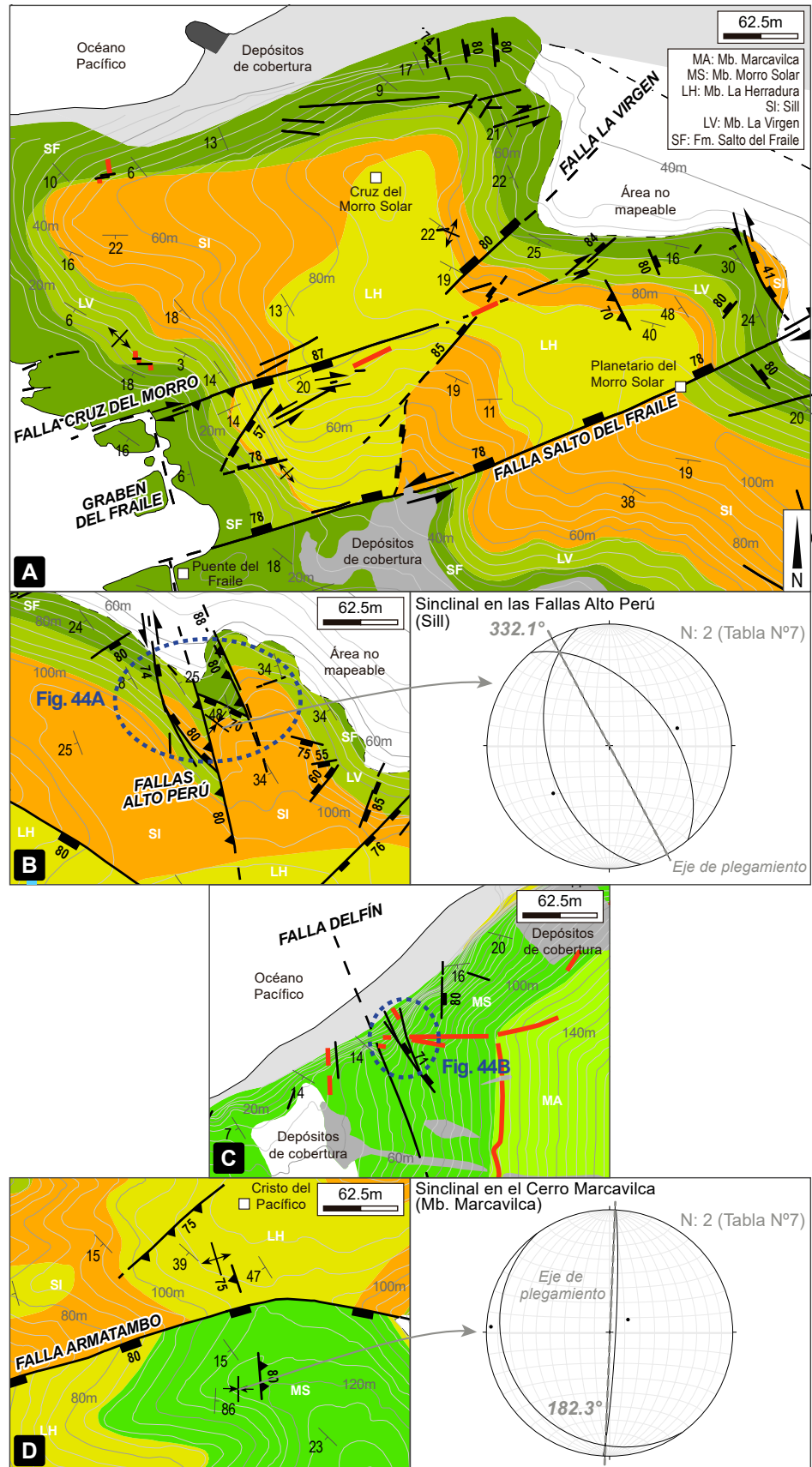
Figura 43. Fallas inversas por compresión en los sectores norte y sur del Morro Solar. Las mediciones de los flancos de los pliegues (N: 4) están descritas en la Tabla N°7. Las líneas rojas corresponden a diques.
