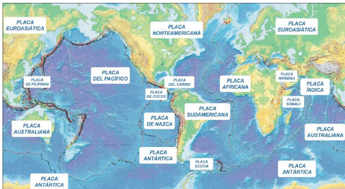
Figura 2. Distribución de las placas tectónicas en la Tierra. Tomado de Simkin et al. (2006).
