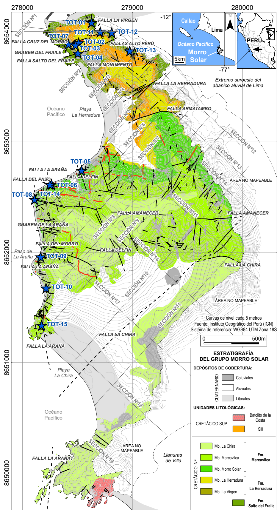
Figura 25. Mapa geológico del Morro Solar a escala 1/5,000 (este trabajo, ver escala más amplia en el Anexo N°1 y en las Tablas de la N°1 a la N°7). Las líneas negras son estructuras tectónicas, las estrellas azules indican la ubicación de estaciones microestructurales (ver datos en las Tablas N°8, N°9 y N°10) y las líneas punteadas corresponden a 19 secciones estructurales (Anexos N°2 y N°3).
