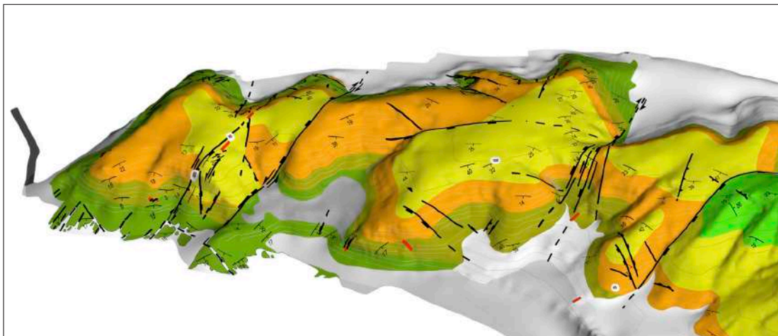
Figura 18. Etapa inicial del modelamiento estructural del sector norte del Morro Solar usando los softwares Blender y Photoshop®.
