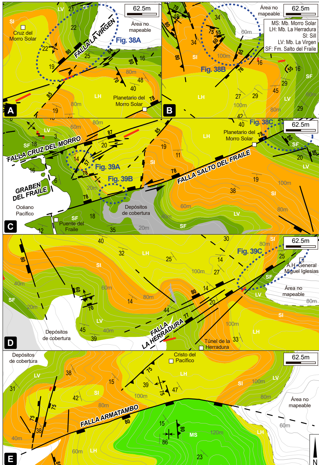
Figura 36. Estructuras extensionales NE-SO/O-E en el sector norte del Morro Solar. Las líneas rojas corresponden a diques.
