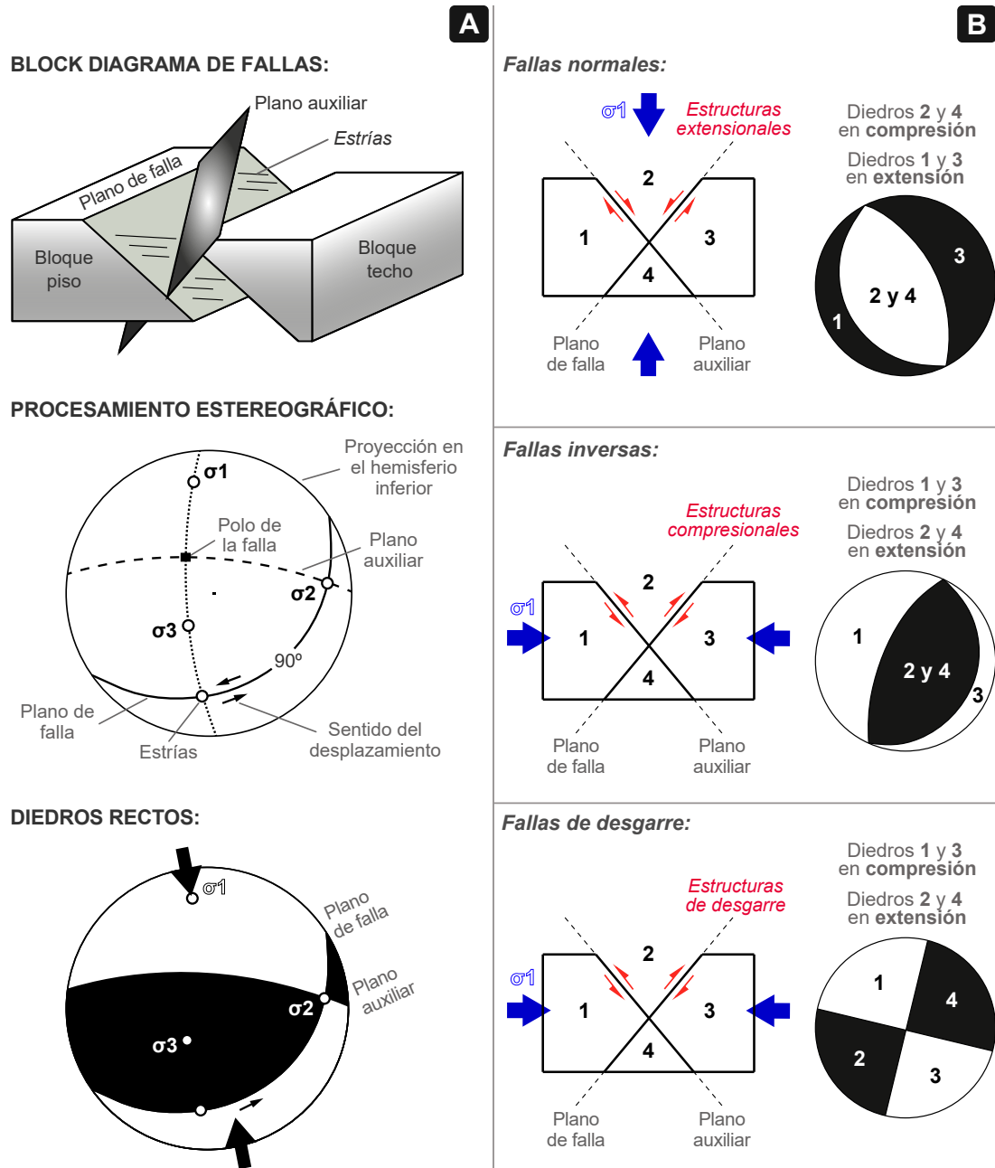
Figura 17. A: Método de los Diedros Rectos empleado para el análisis estructural dinámico de fallas. B: Las mejores interpretaciones se obtienen utilizando los modelos de Anderson (1905 y 1951) y de Ramsay (1967). Tomado de Allmendinger (1987).
