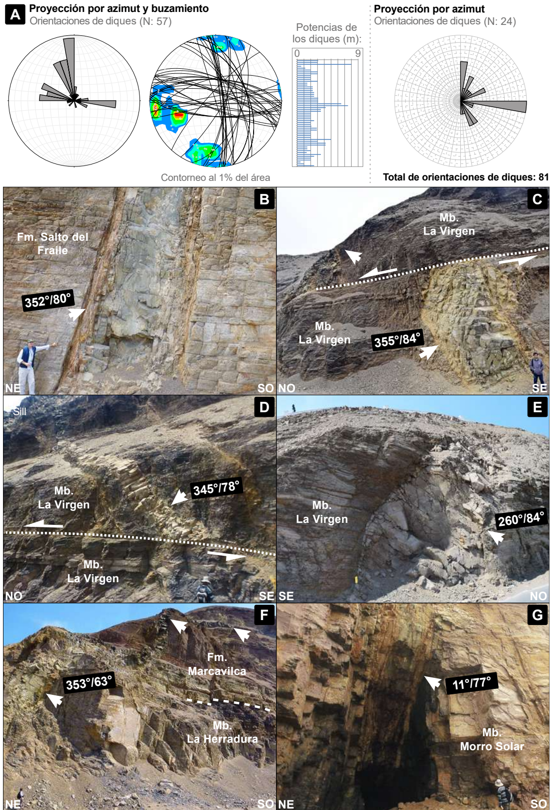
Figura 30. Orientaciones de diques (N: 81). 57 mediciones se obtuvieron en campo y 24 azimuts se extrajeron de la fotointerpretación geológica pre y poscampo (ver Tabla N°1). La ubicación de los diques está señalada por las flechas blancas. “N” representa el número de datos medidos.
