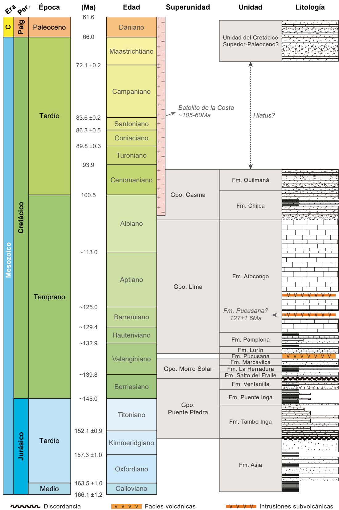
Figura 21. Estratigrafía del antearco peruano de la región Lima, sintetizada partir de los trabajos de Palacios et al. (1992), Romero et al. (2005), Aleman et al. (2006), Romero (2007) y Jacay et al. (2015). Tiempo geológico según Cohen et al. (2013).
