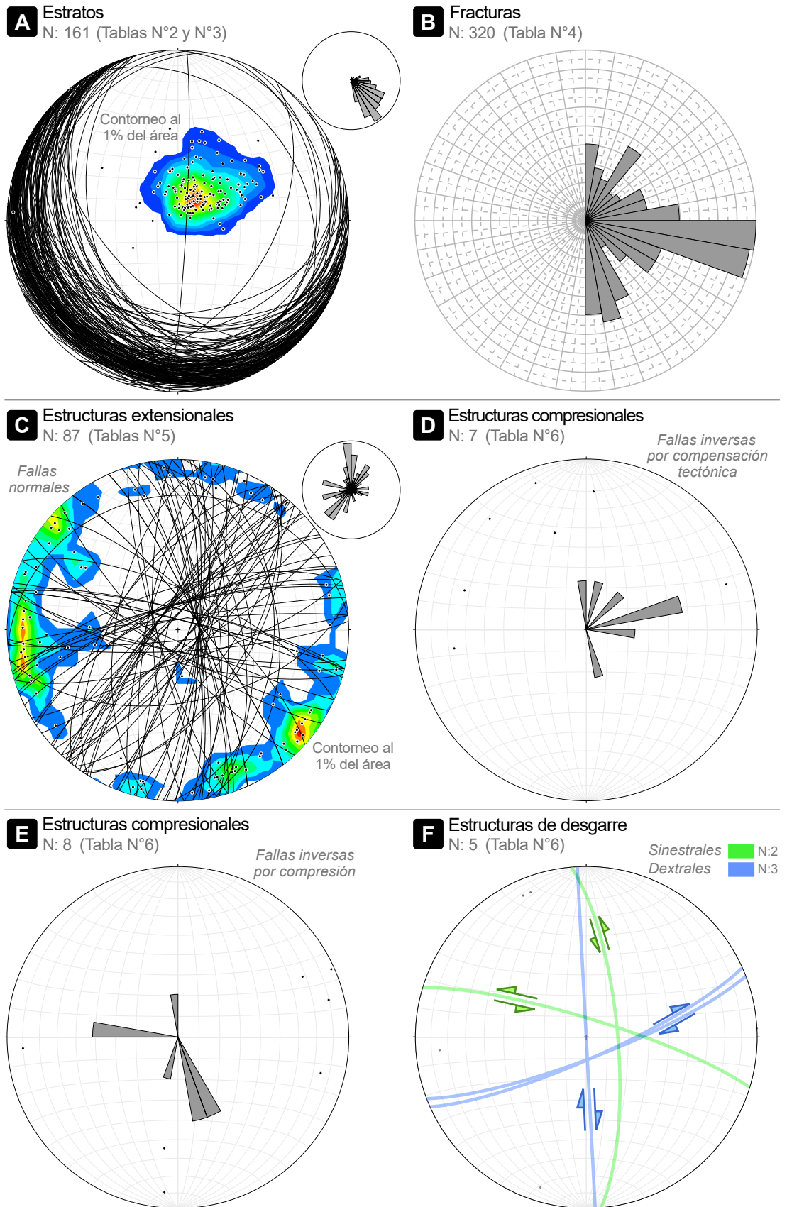
Figura 31. Mediciones estructurales en el Morro Solar (ver Tablas N°2, N°3, N°4, N°5 y N°6). “N” representa el número de datos medidos.
