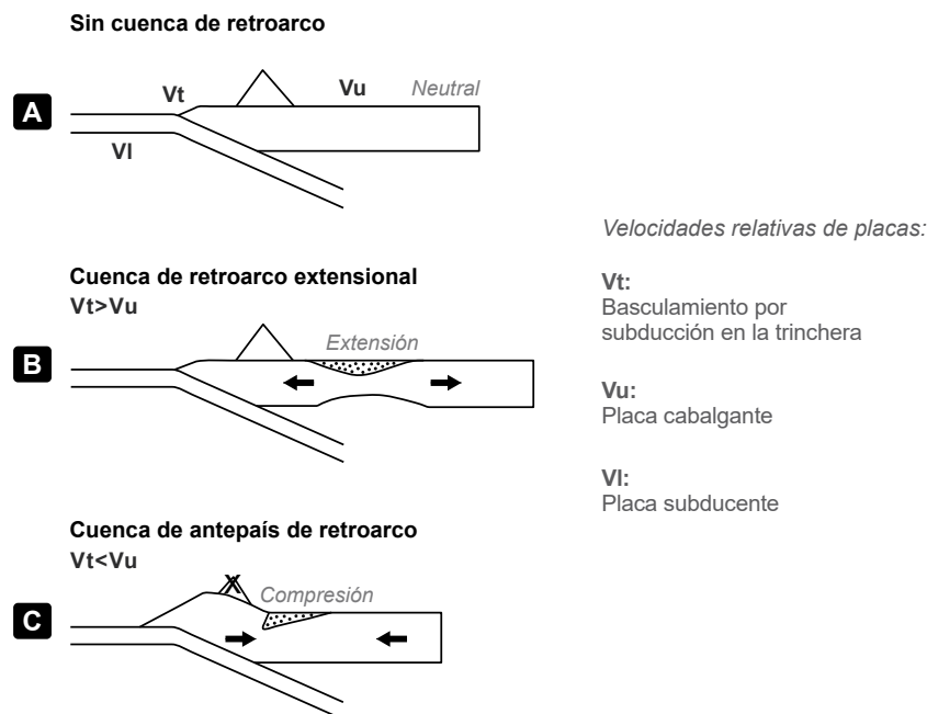
Figura 5. Velocidades de convergencia de placas y sus efectos en la placa tectónica cabalgante. Tomado de Daly (1989) y Royden (1993).
