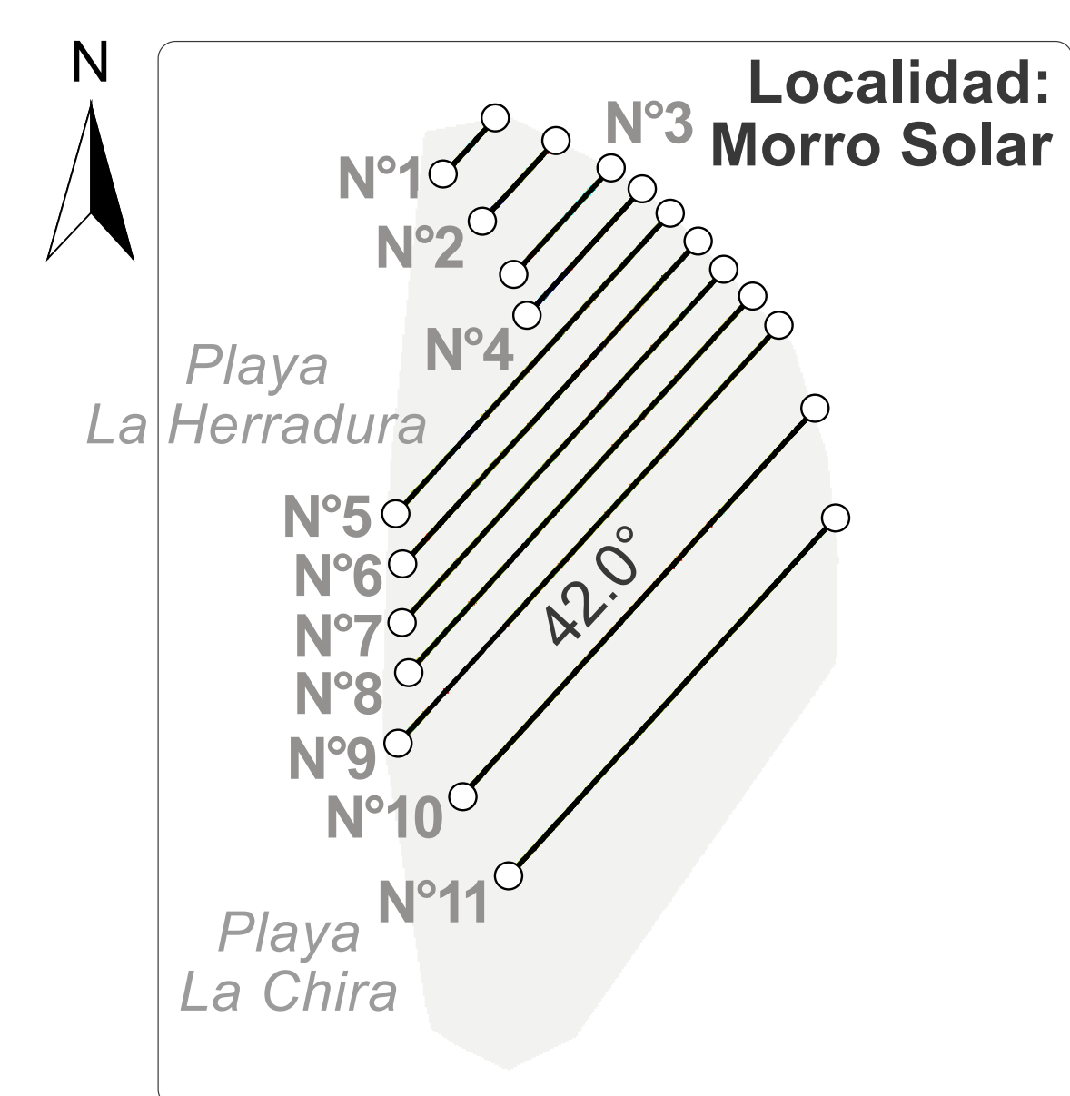
SECCIONES ESTRUCTURALES SO-NE
