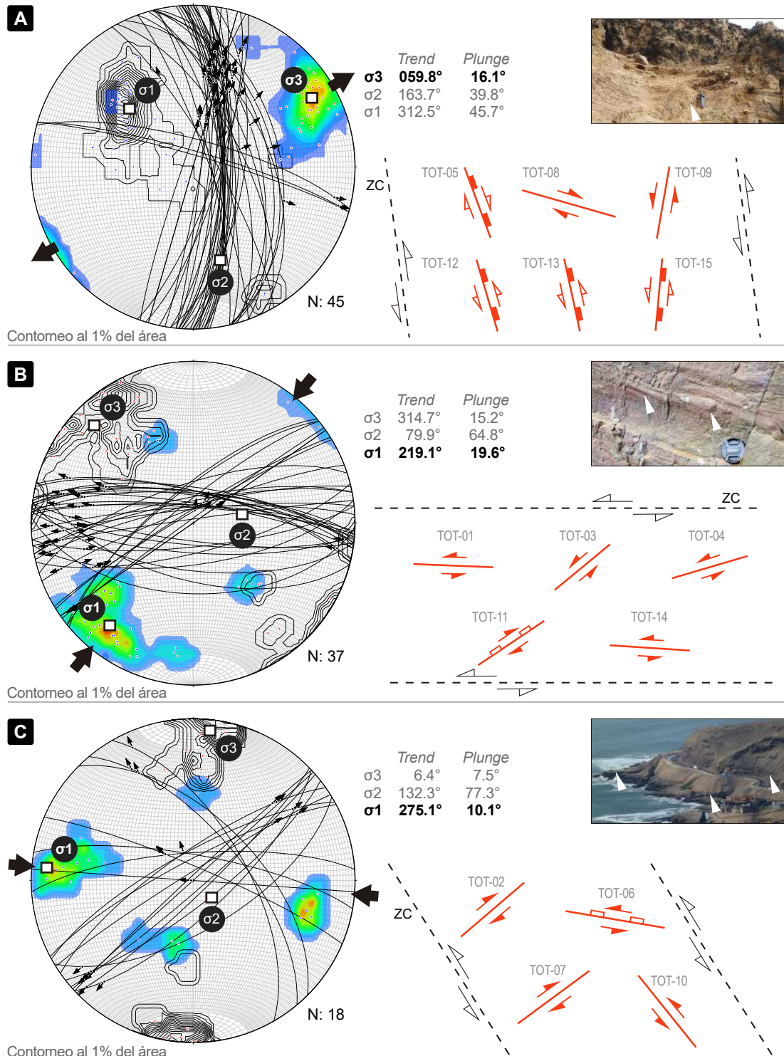
Figura 46. Estados de paleoesfuerzos asociados a las estructuras mesoscópicas y microestructuras tectónicas del Morro Solar (ver datums de falla en las Tablas N°8, N°9 y N°10). ZC: Zona de cizalla principal.
