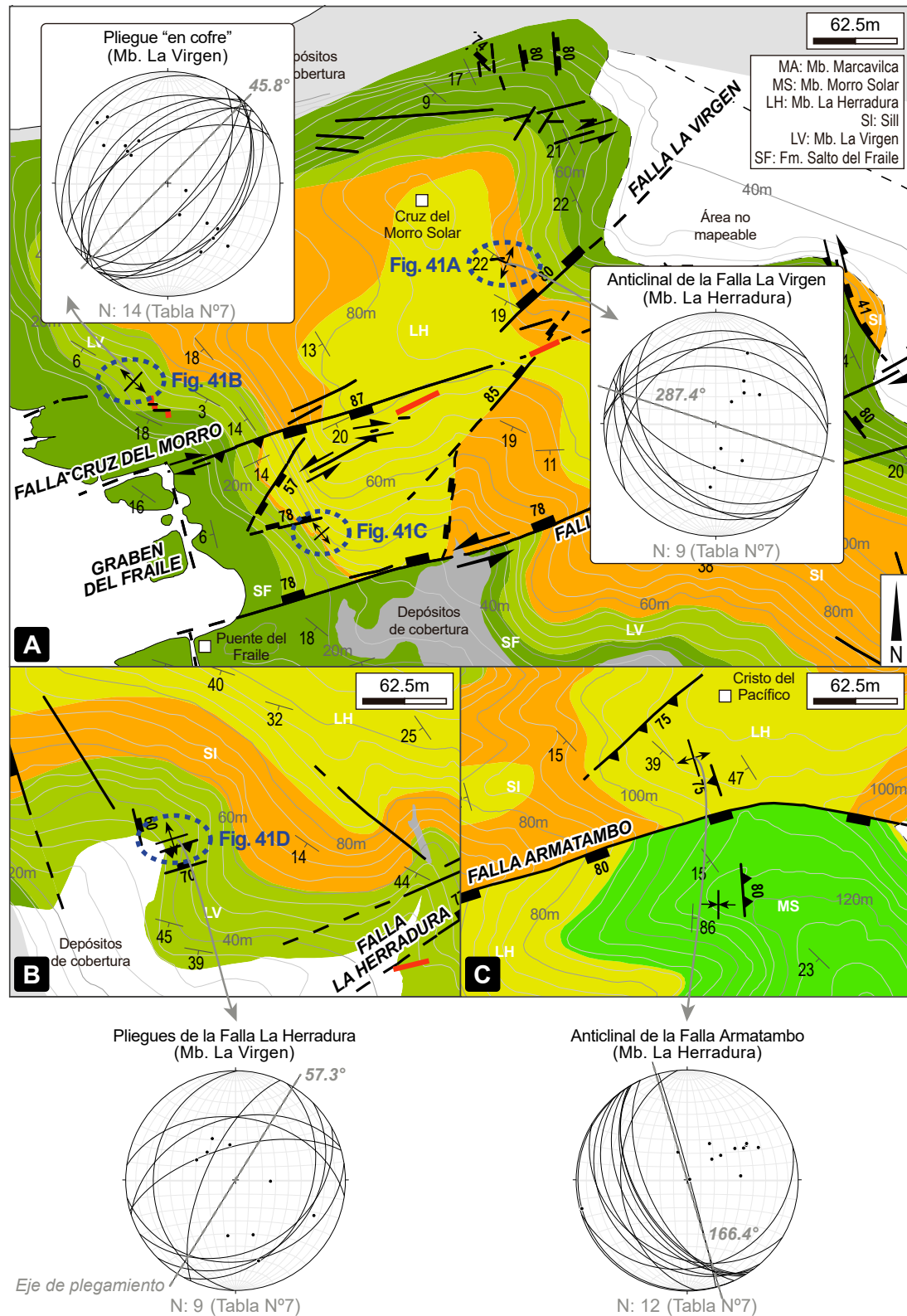
Figura 40. Pliegues y fallas inversas por compensación tectónica en el sector norte del Morro Solar. Las mediciones de los flancos de pliegues (N: 44) están descritas en la Tabla N°7. Las líneas rojas corresponden a diques.
