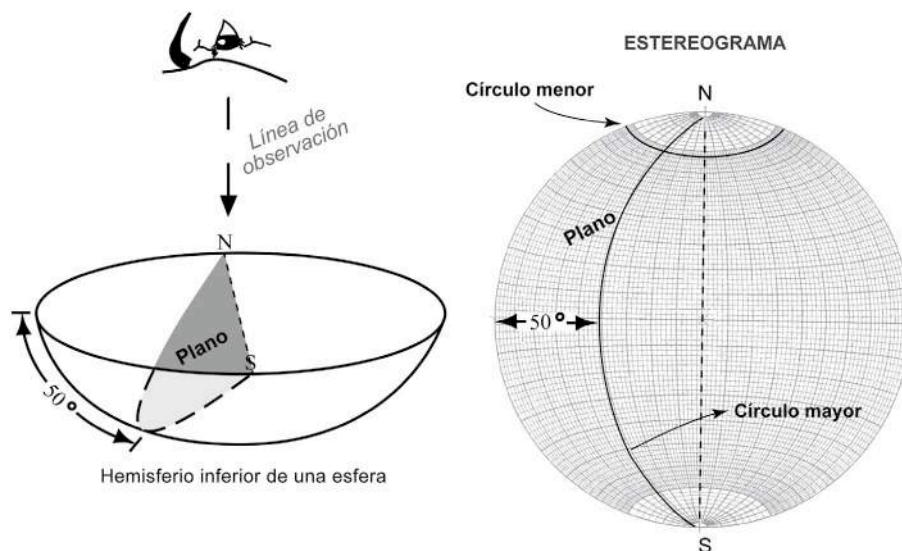
Figura 16. Estereofalsilla de Schmidt. Tomado de Rowland et al. (2007).
