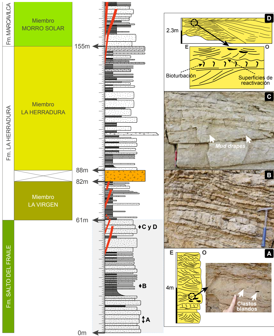
Figura 27. Columna estratigráfica de la Formación Salto del Fraile.
