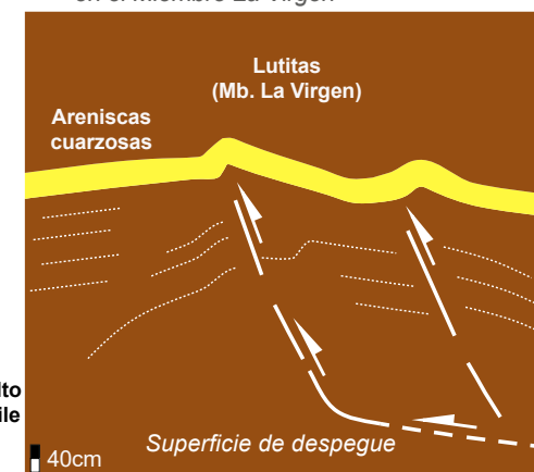
C Pliegues de la Falla La Herradura en el Miembro La Virgen
