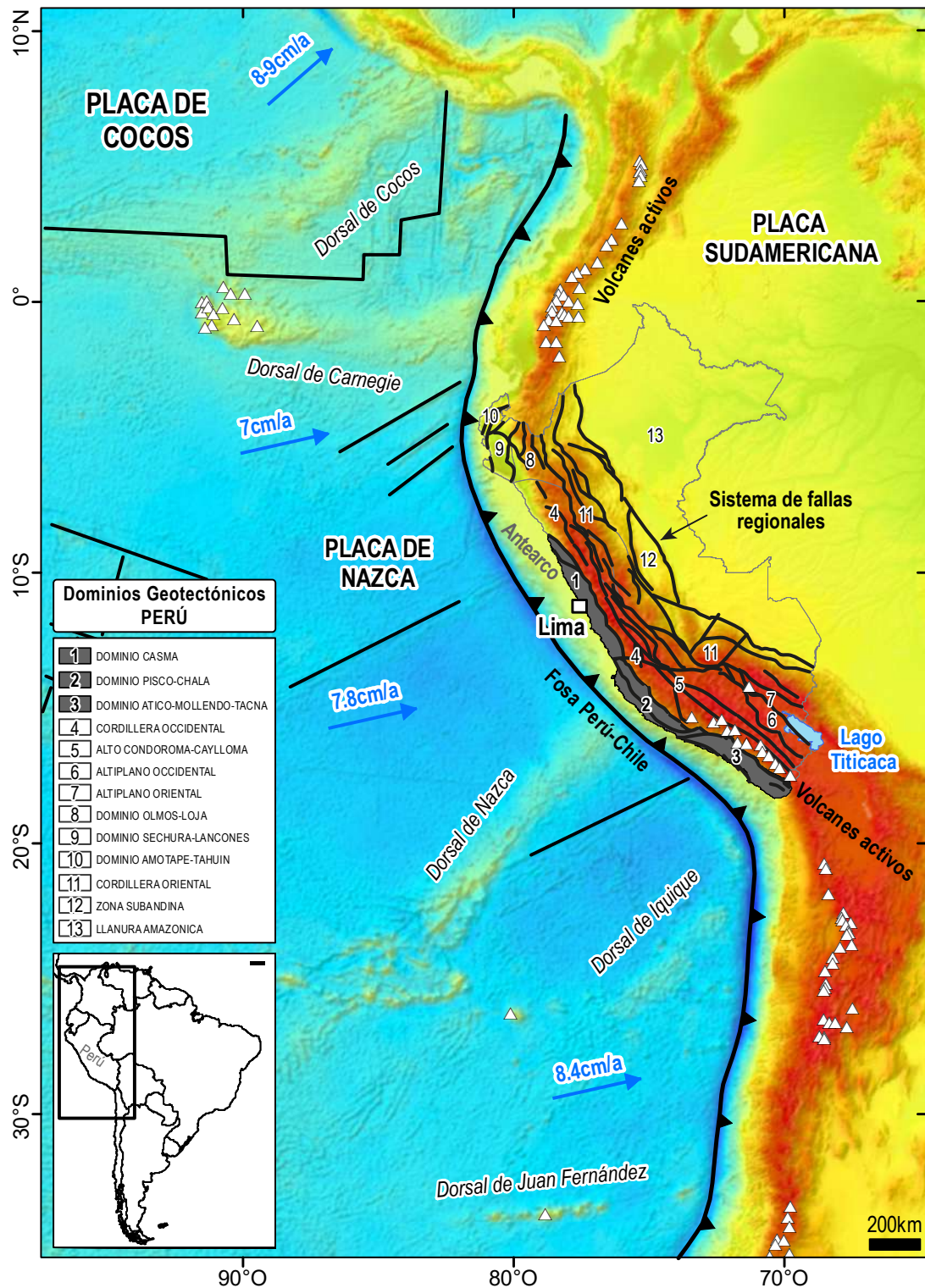
Figura 1. El antearco peruano se encuentra en el extremo oeste de la Cordillera Occidental y está conformado por los dominios geotectónicos: 1 (Casma), 2 (Pisco-Chala) y 3 (Atico-Mollendo-Tacna). Tomado y basado de Carlotto et al. (2009) y Sébrier et al. (1988).
