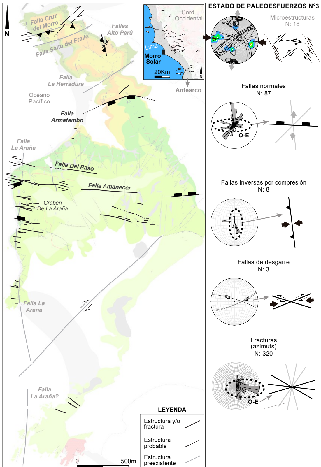
Figura 53. Estado de paleoesfuerzos N°3 en el Morro Solar. Está asociado a una compresión O-E que produjo fallas normales O-E, fallas inversas junto con pliegues menores N-S y fallas de desgarre NO-SE/NE-SO.
