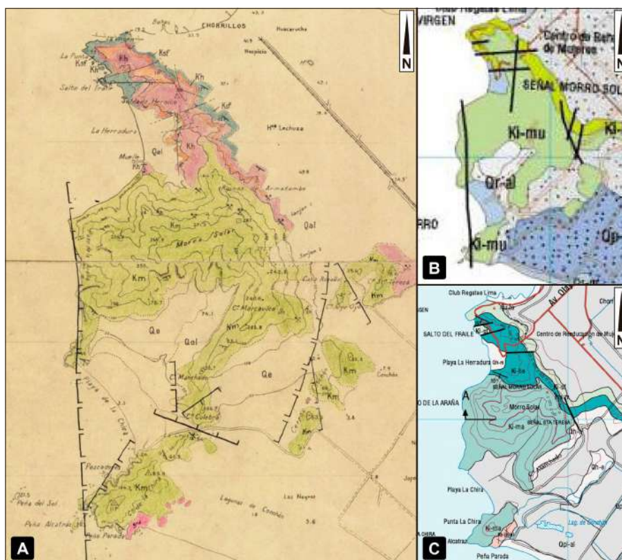
Figura 24. Cartografía geológica clásica del Morro Solar. Tomado de A: Fernández et al. (1958), B: Caldas y Palacios (1998) y C: León y De La Cruz (2002).
