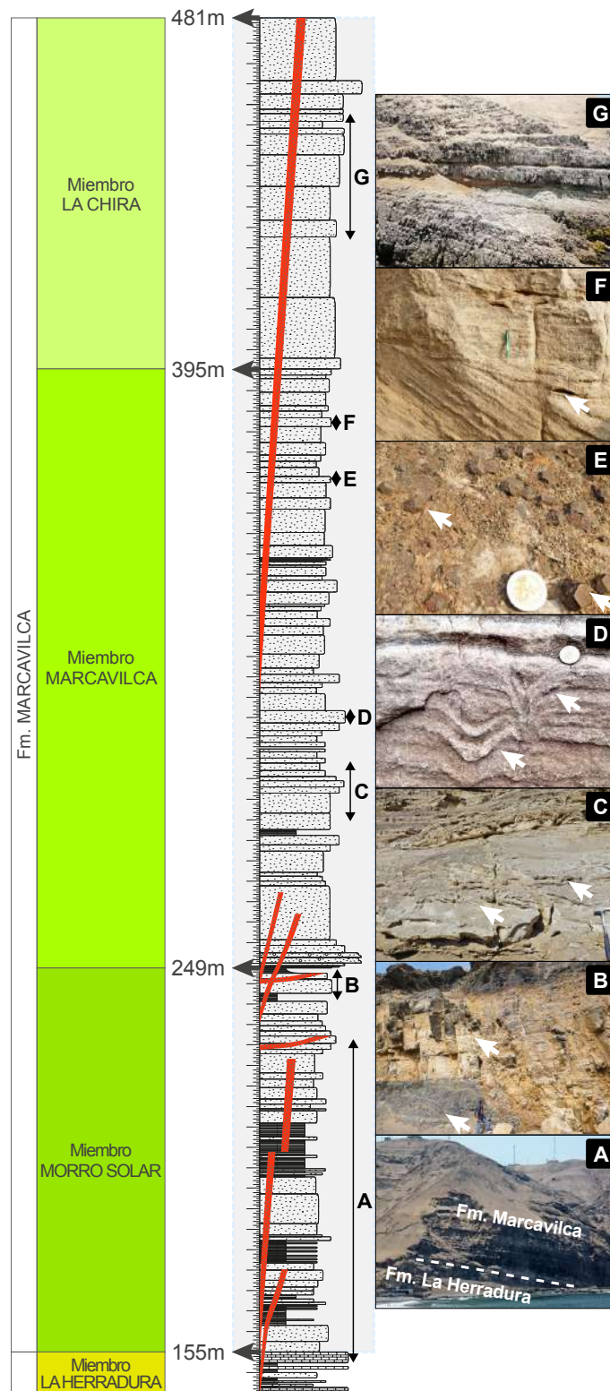
Figura 29. Columna estratigráfica de la Formación Marcavilca.
