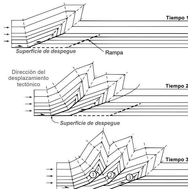
Figura 11. Arquitectura tectónica de fallas inversas y pliegues (Suppe y Donald, 1990; Erslev, 1991). Tomado de Van Der Pluijm y Marshak (2004).
