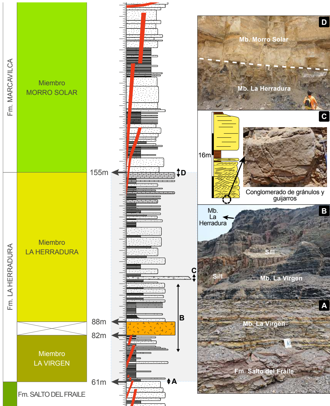
Figura 28. Columna estratigráfica de la Formación La Herradura.
