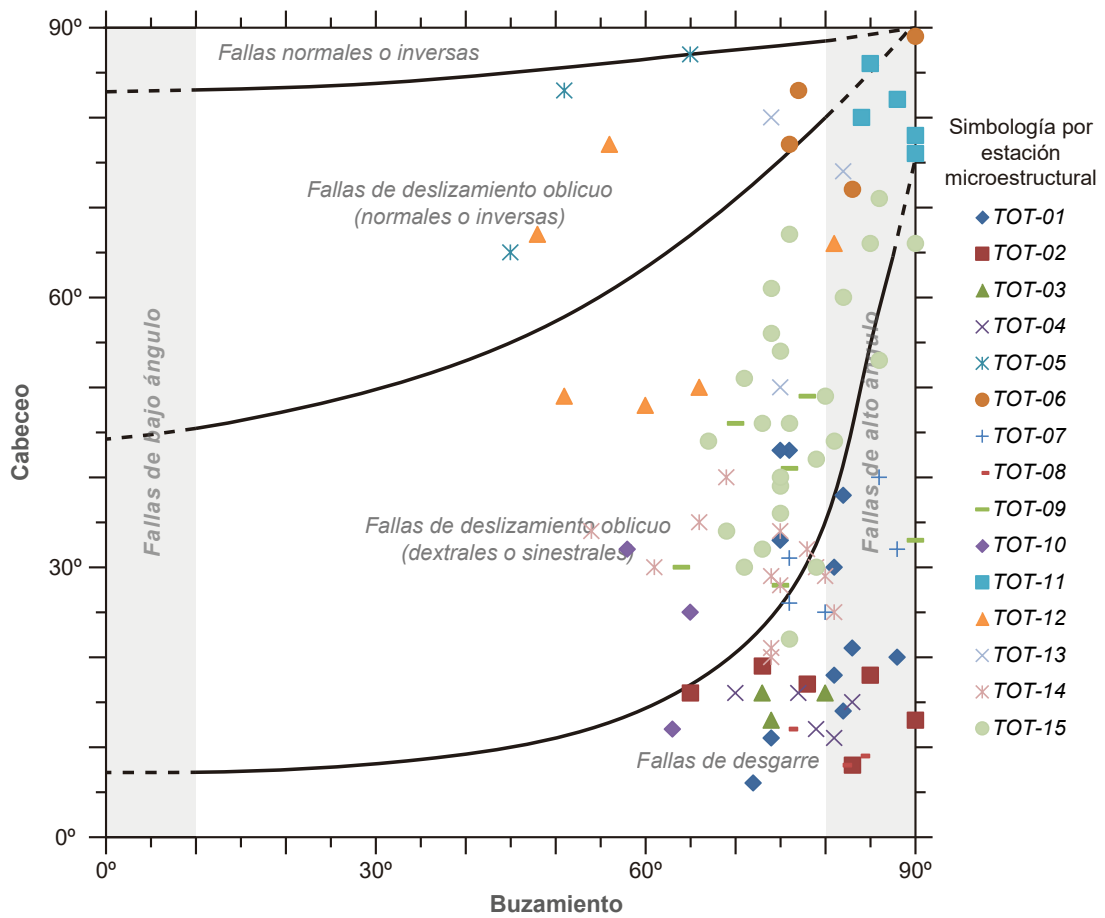
Figura 45. Cinemáticas de las microestructuras tectónicas del Morro Solar según la clasificación de fallas de Angelier (1994). Los datums de falla están descritos en las Tablas N°8, N°9 y N°10.
