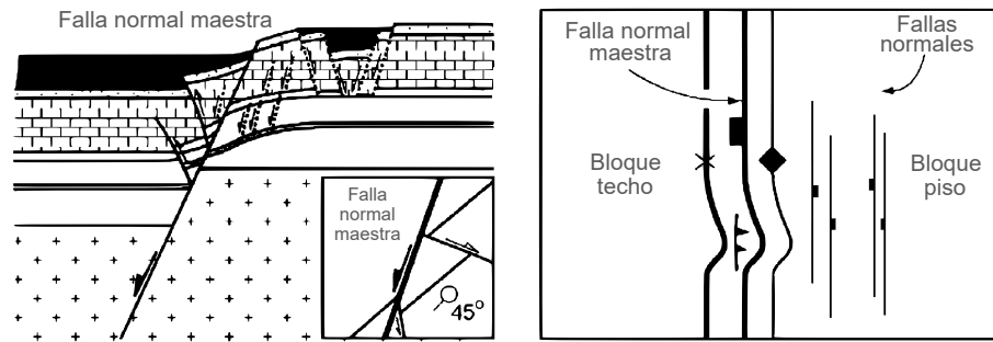
Figura 10. Arquitectura tectónica de fallas normales (Peacock et al., 2000; Delogkos et al., 2017), las fallas inversas tienen lugar por compensación tectónica cerca de reologías dúctiles. Tomado de Jackson et al. (2006).
