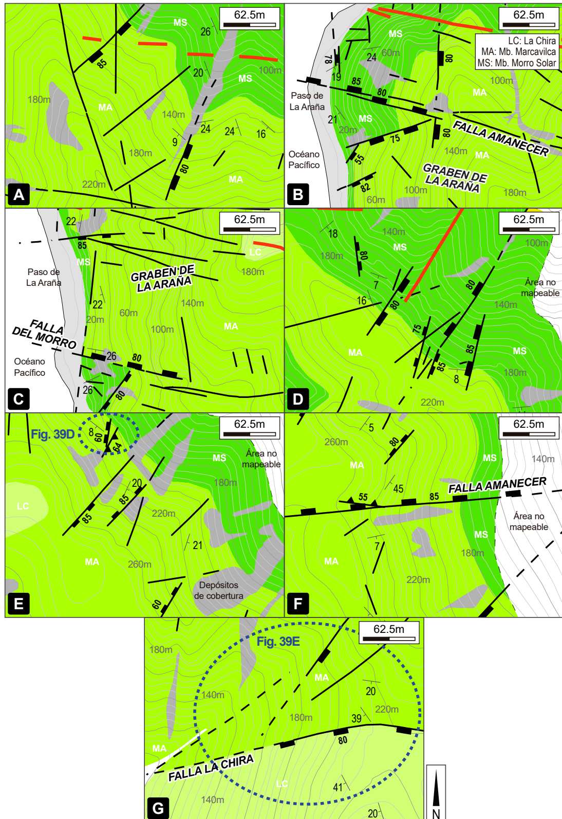
Figura 37. Estructuras extensionales NE-SO/O-E en el sector sur del Morro Solar. Las líneas rojas corresponden a diques.
