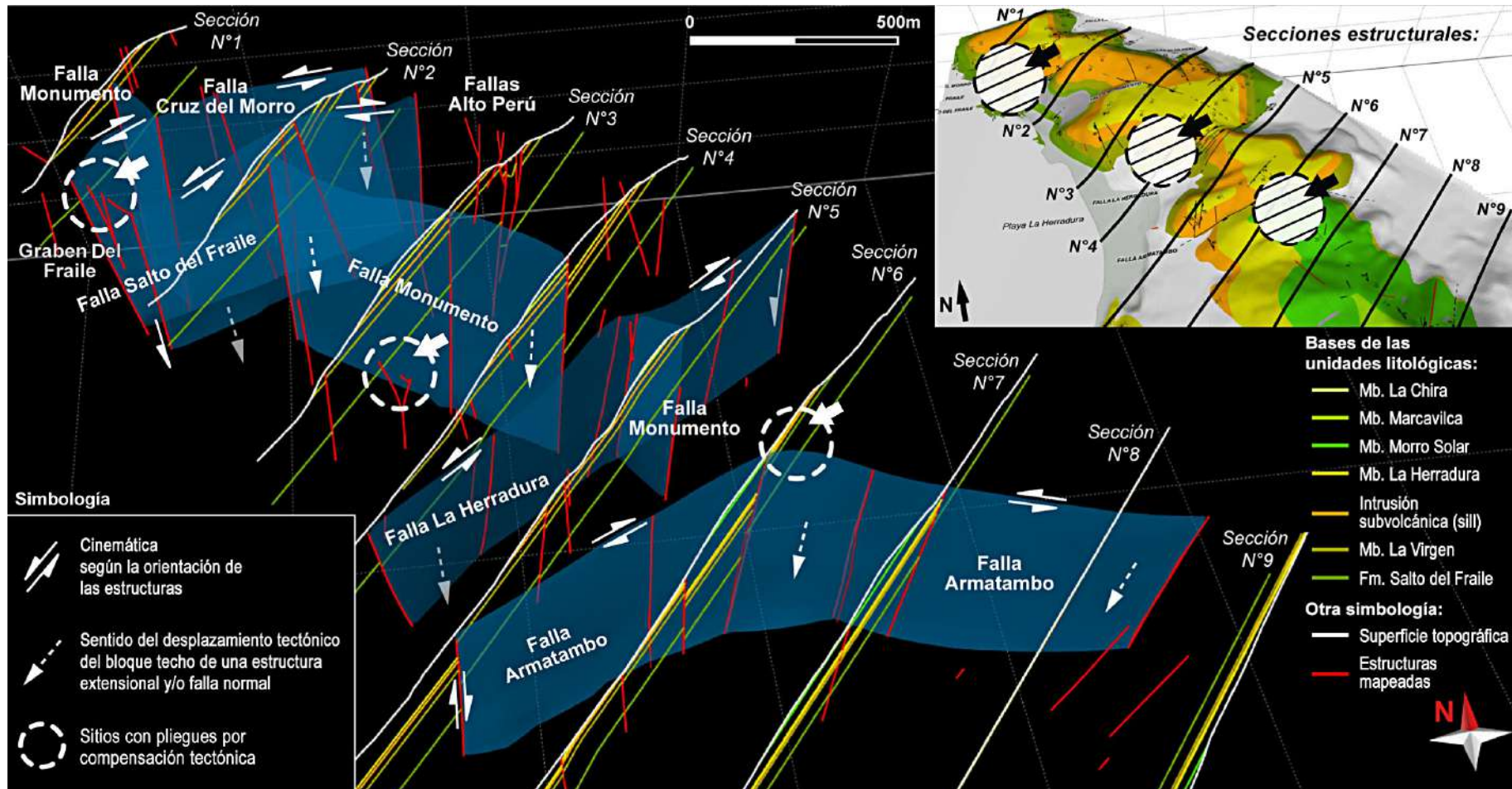
Figura 49. Modelo estructural 3D del sector norte del Morro Solar construido a partir de las secciones SO-NE ( 42.0^\circ ). Las geometrías de las estructuras principales y secundarias están dadas por planos azules y líneas rojas, respectivamente.
