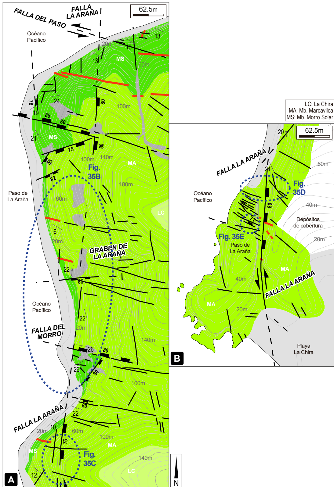
Figura 33. Estructuras extensionales N-S/NO-SE en el sector sur del Morro Solar. Las líneas rojas corresponden a diques.
