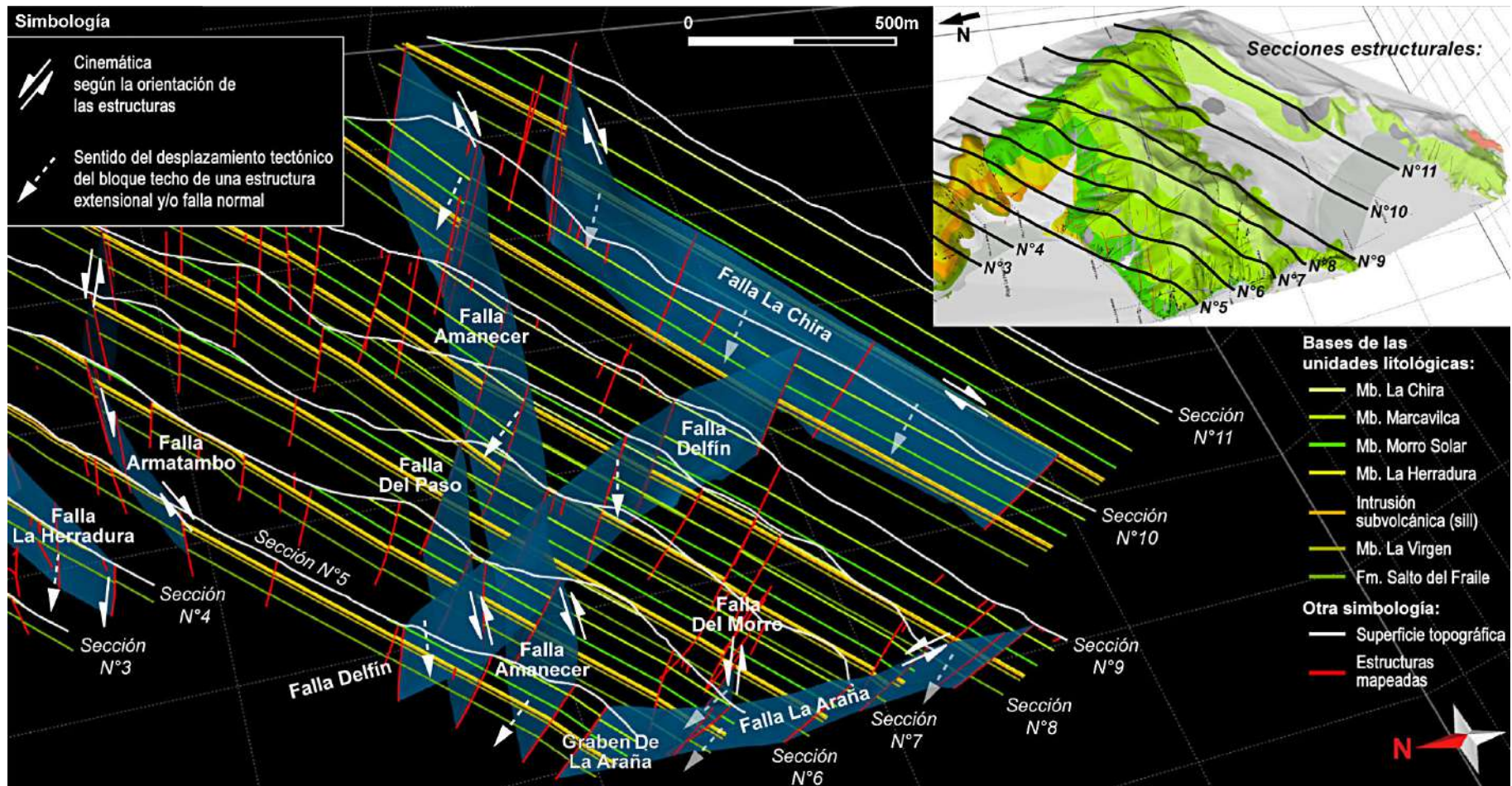
Figura 50. Modelo estructural 3D del sector sur del Morro Solar construido a partir de las secciones SO-NE (42.0°). Las geometrías de las estructuras principales y secundarias están dadas por planos azules y líneas rojas, respectivamente.
