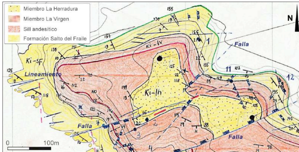
Figura 14. Etapa inicial del mapeo geológico de campo (sector norte del Morro Solar).
