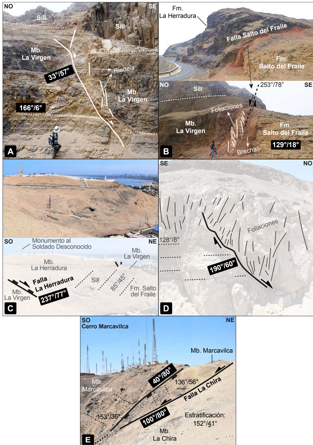
Figura 39. Vistas de campo del mapeo geológico observado en las Figuras 36 y 37.
