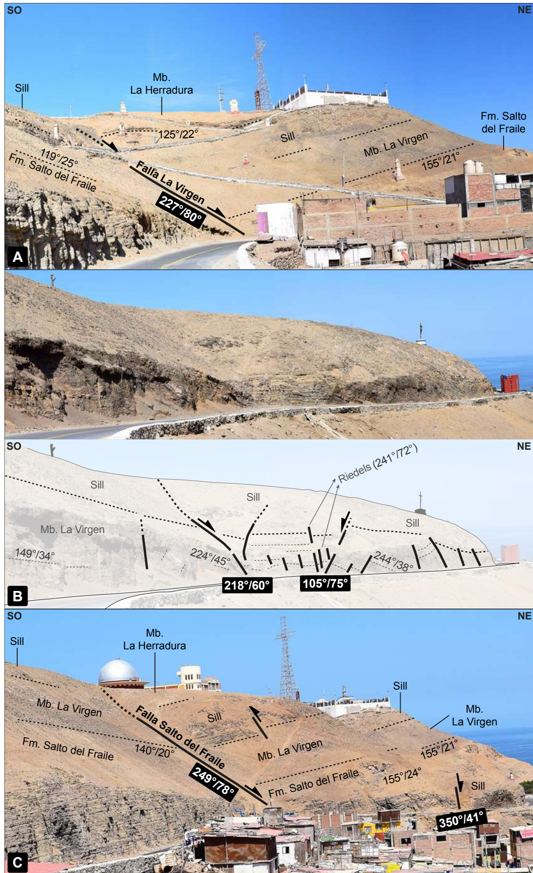
Figura 38. Vistas de campo del mapeo geológico observado en la Figura 36.
