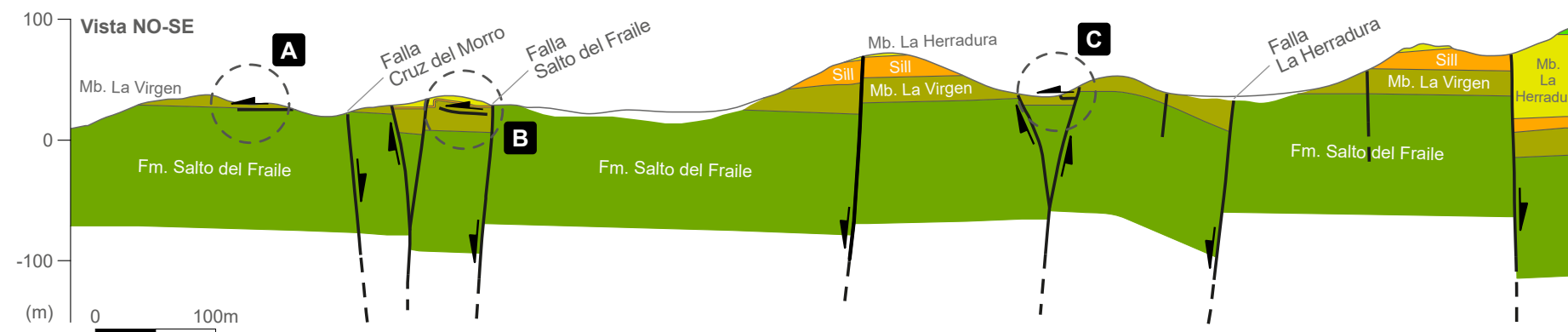
B Anticlinal volcado en sill adyacente a la Falla Salto del Fraile
