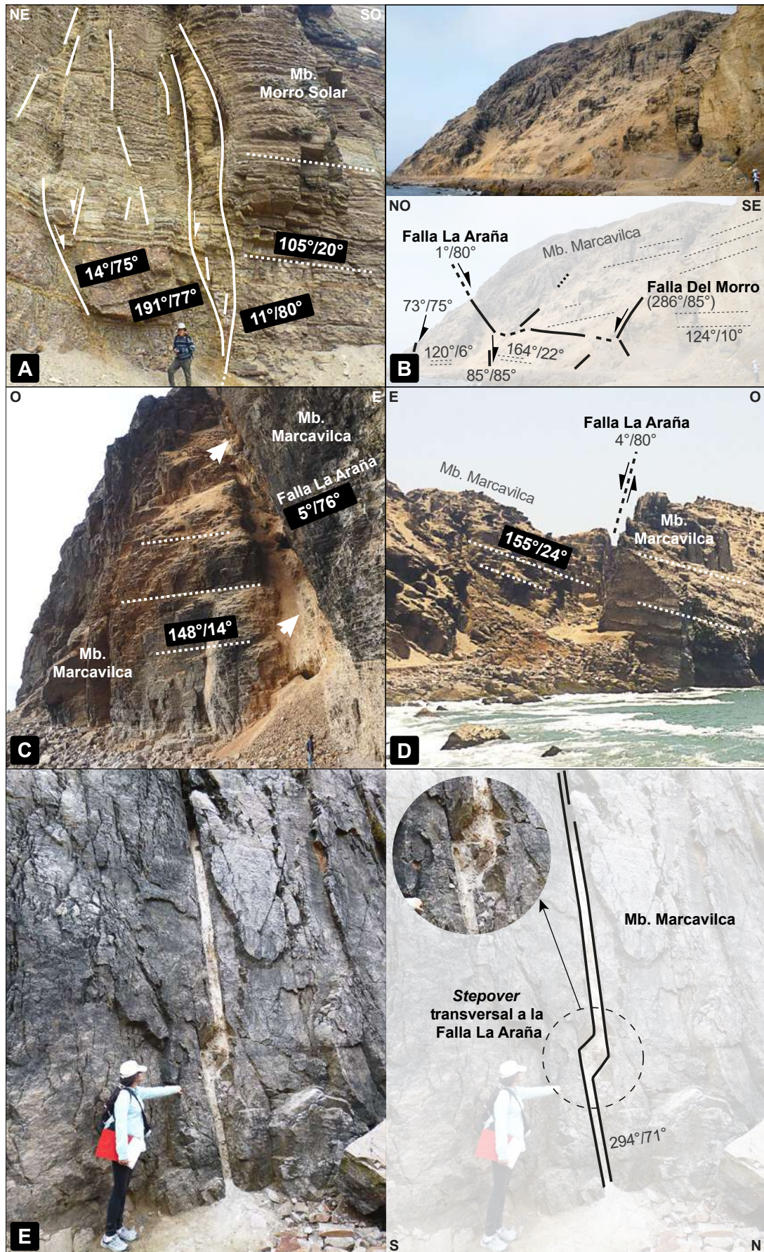
Figura 35. Vistas de campo del mapeo geológico observado en las Figuras 32 y 33.
