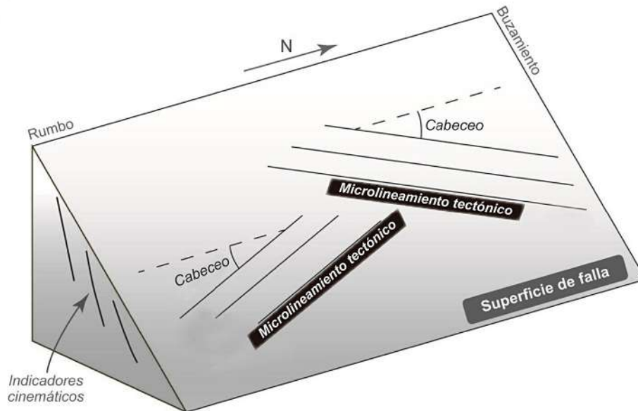
Figura 15. Bloque-diagrama de los datums de falla tomados en una estación microestructural. Basado y modificado de Rowland et al. (2007).
