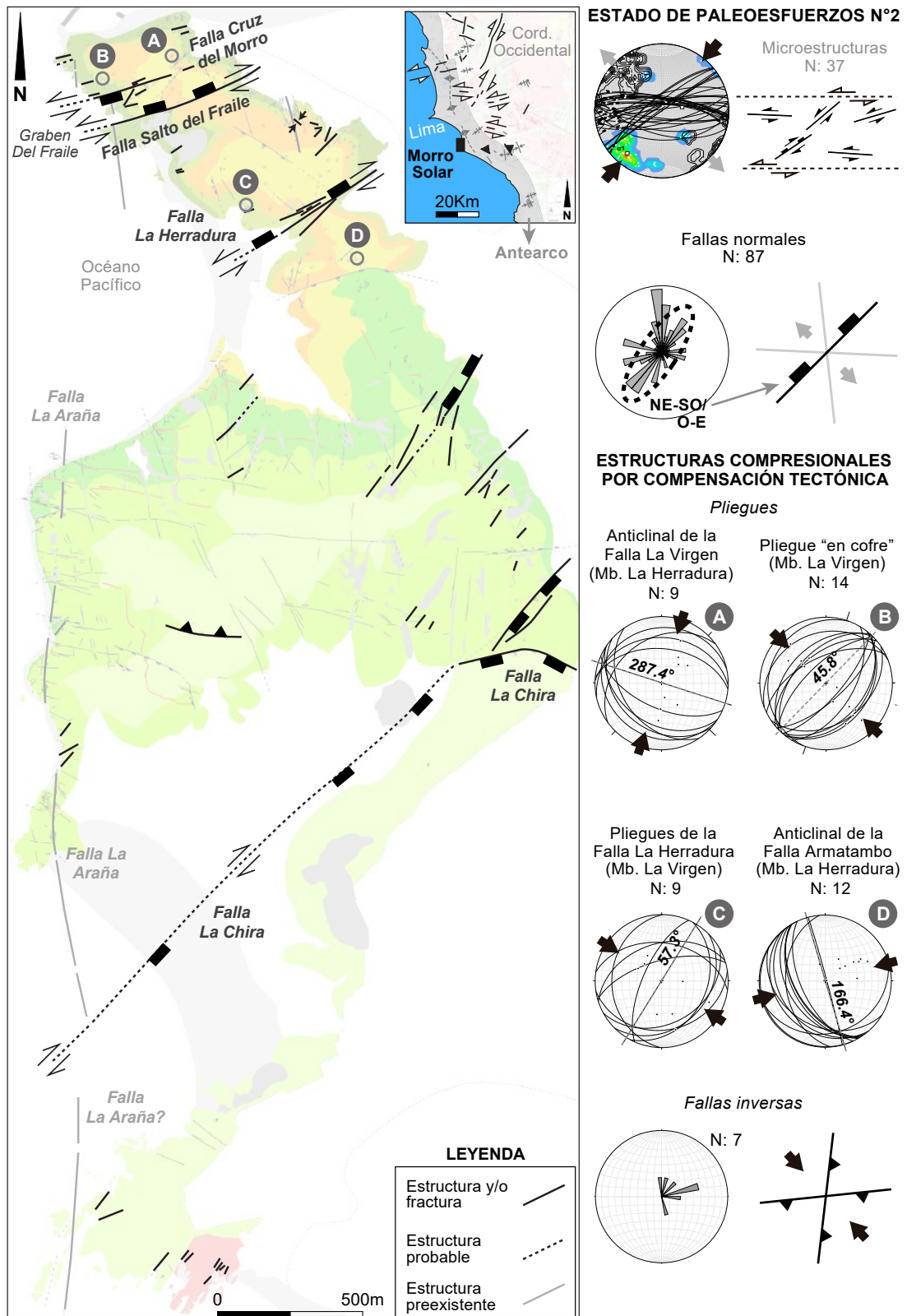
Figura 52. Estado de paleoesfuerzos N°2 en el Morro Solar. Está asociado a una compresión NE-SO que produjo fallas normales, pliegues y fallas inversas NE-SO/O-E (por compensación tectónica).
