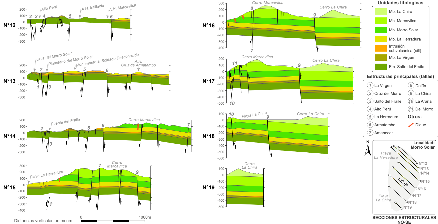
Figura 48. Secciones estructurales NO-SE de azimuth 132.6° en el Morro Solar (ver escala más amplia en el Anexo N°3). Sus longitudes en kilómetros son: N°12=1.62, N°13=2.21, N°14=2.56, N°15=1.94, N°16=2.09, N°17=1.98, N°18=1.59 y N°19=0.57.
