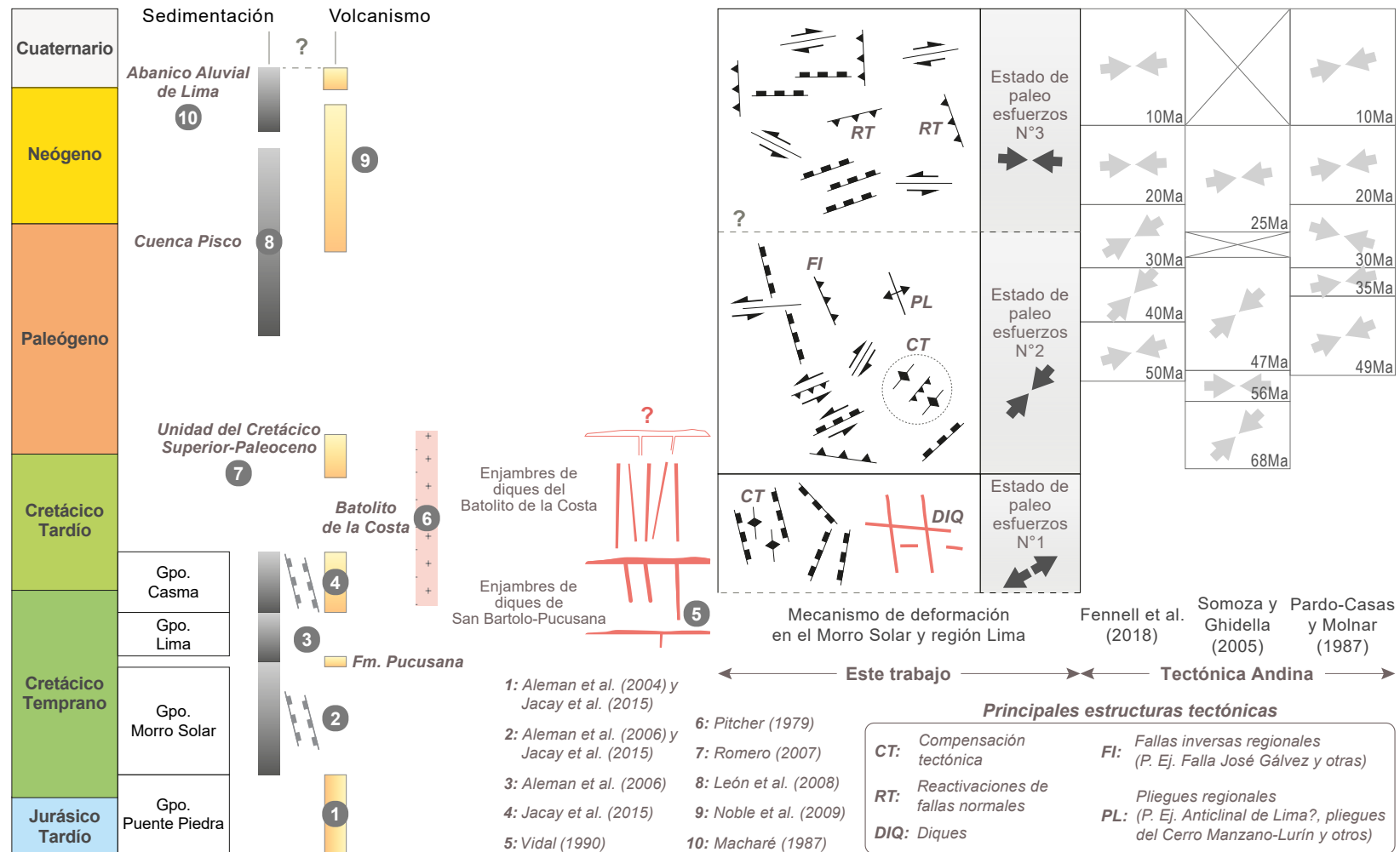
Figura 54. Evolución tectónica del mecanismo de deformación del Morro Solar. Esta interpretación se propone tentativamente comparando los estados de paleoesfuerzos del Morro Solar y las convergencias de placas en el margen occidental andino durante el Cenozoico.
