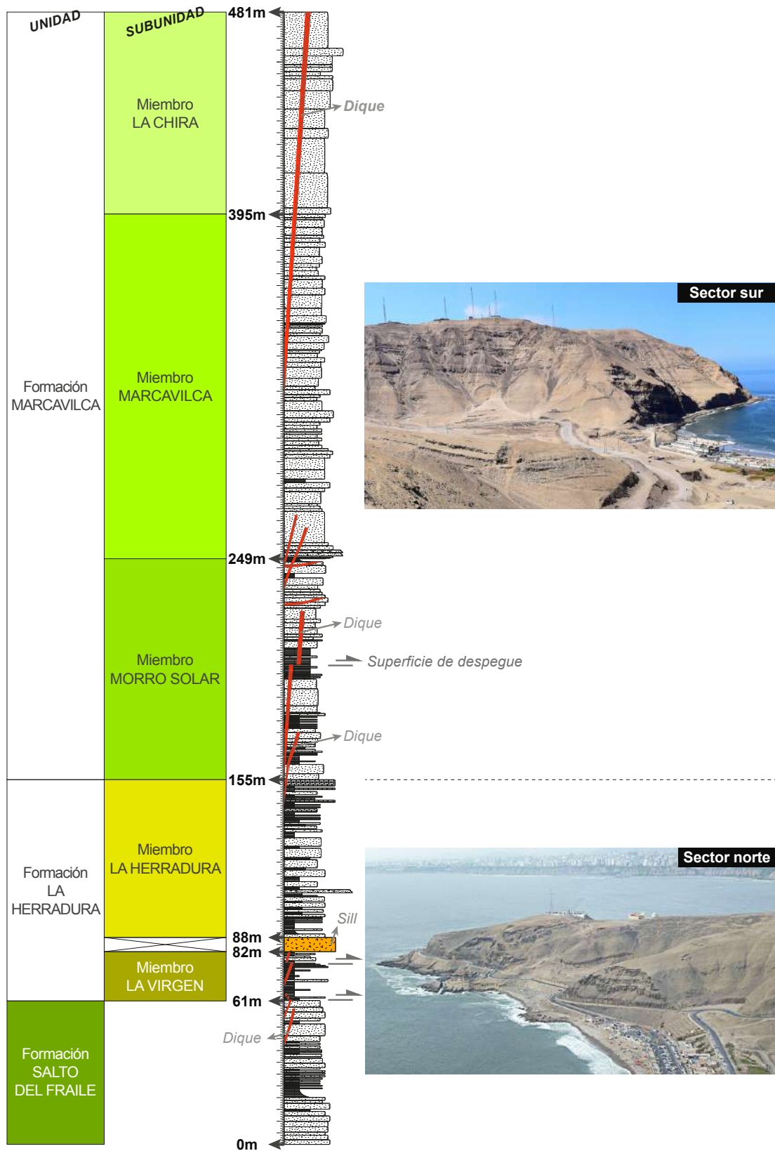
Figura 26. Estratigrafía del Grupo Morro Solar levantada cada 5 m en el área de estudio (ver a escala 1/1,200 en el Anexo N°1).
