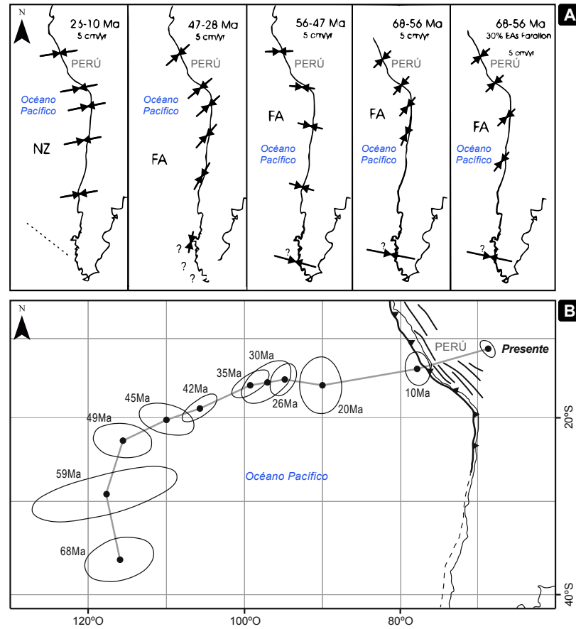
Figura 4. A: Convergencia de las placas Farallón (FA)-Sudamericana (68-28 Ma) y Nazca (NZ)-Sudamericana (26-10 Ma). B: Durante el Cenozoico, los vectores de convergencia de placas tuvieron direcciones NE-SO y O-E. Tomado de Somoza y Ghidella (2005) y Pardo-Casas y Molnar (1987).
