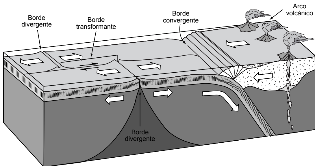
Figura 3. Movimientos y tipos de bordes de las placas tectónicas en los Andes. Tomado de Van Der Pluijm y Marshak (2004).
