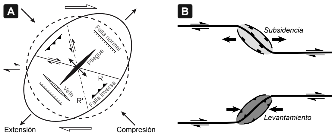
Figura 13. A: Modelo de Ramsay (1967). B: Deformación tectónica transtensional (subsidencia) y transpresional (levantamiento). Tomado de Van Der Pluijm y Marshak (2004) y McClay y Bonora (2001).
