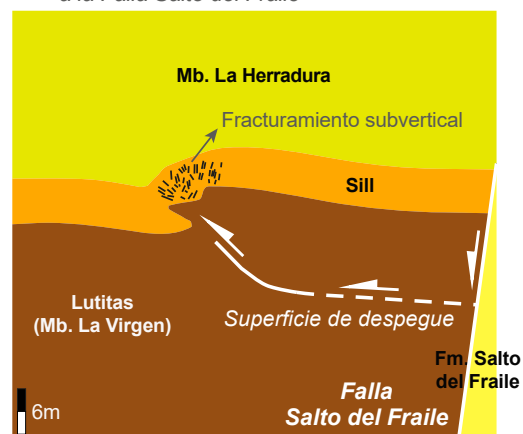
B Anticlinal volcado en sill adyacente a la Falla Salto del Fraile
