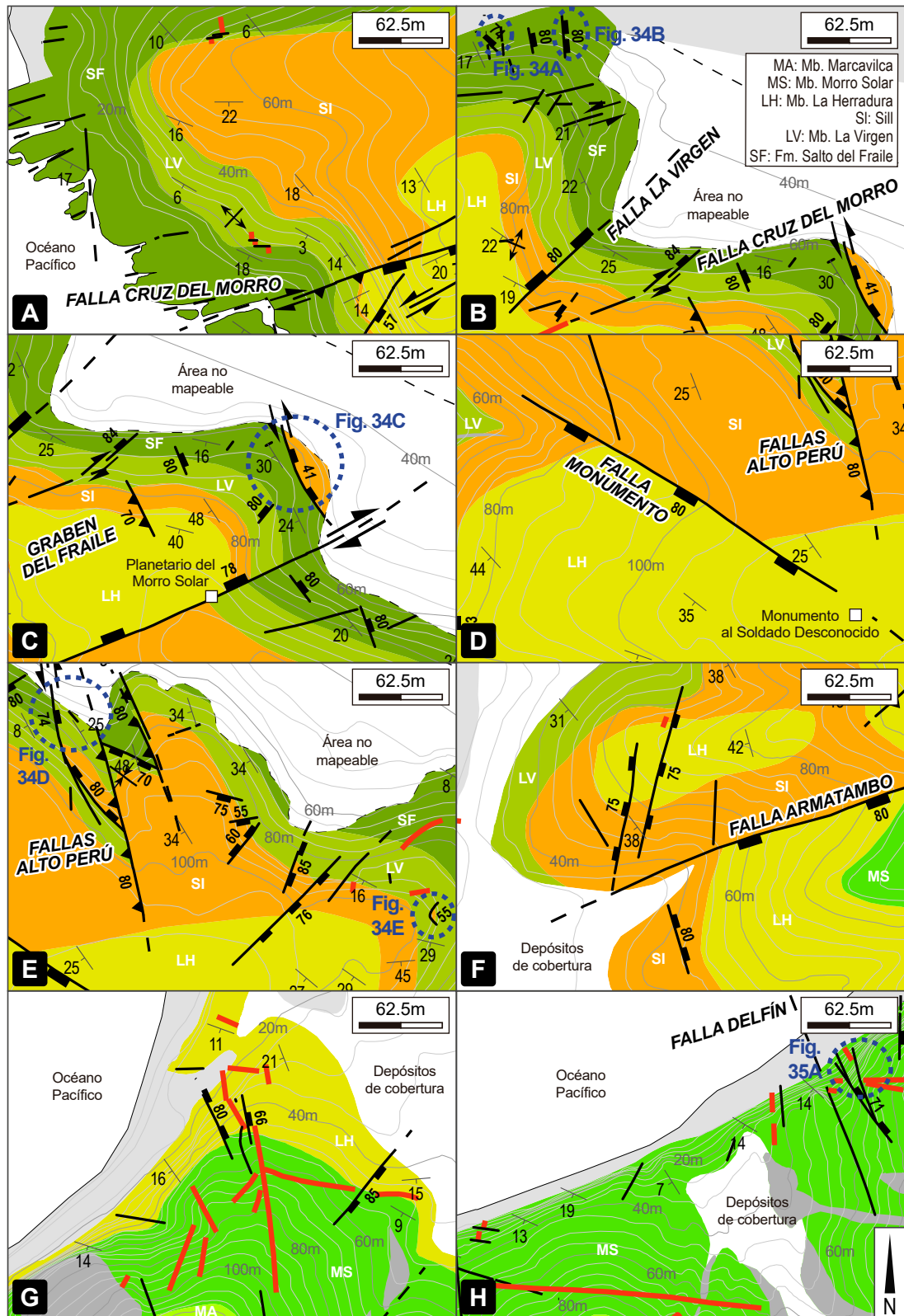
Figura 32. Estructuras extensionales N-S/NO-SE en el sector norte del Morro Solar. Las líneas rojas corresponden a diques.
