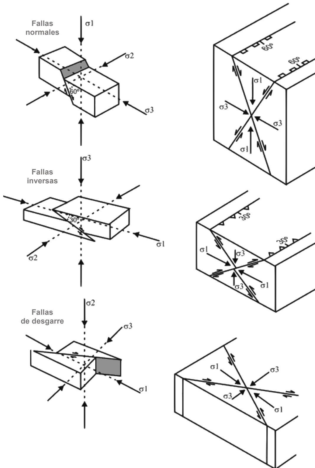
Figura 9. Cinemáticas de estructuras tectónicas asociadas a estados de esfuerzos según el modelo dinámico de fallas de Anderson (1905 y 1951).
