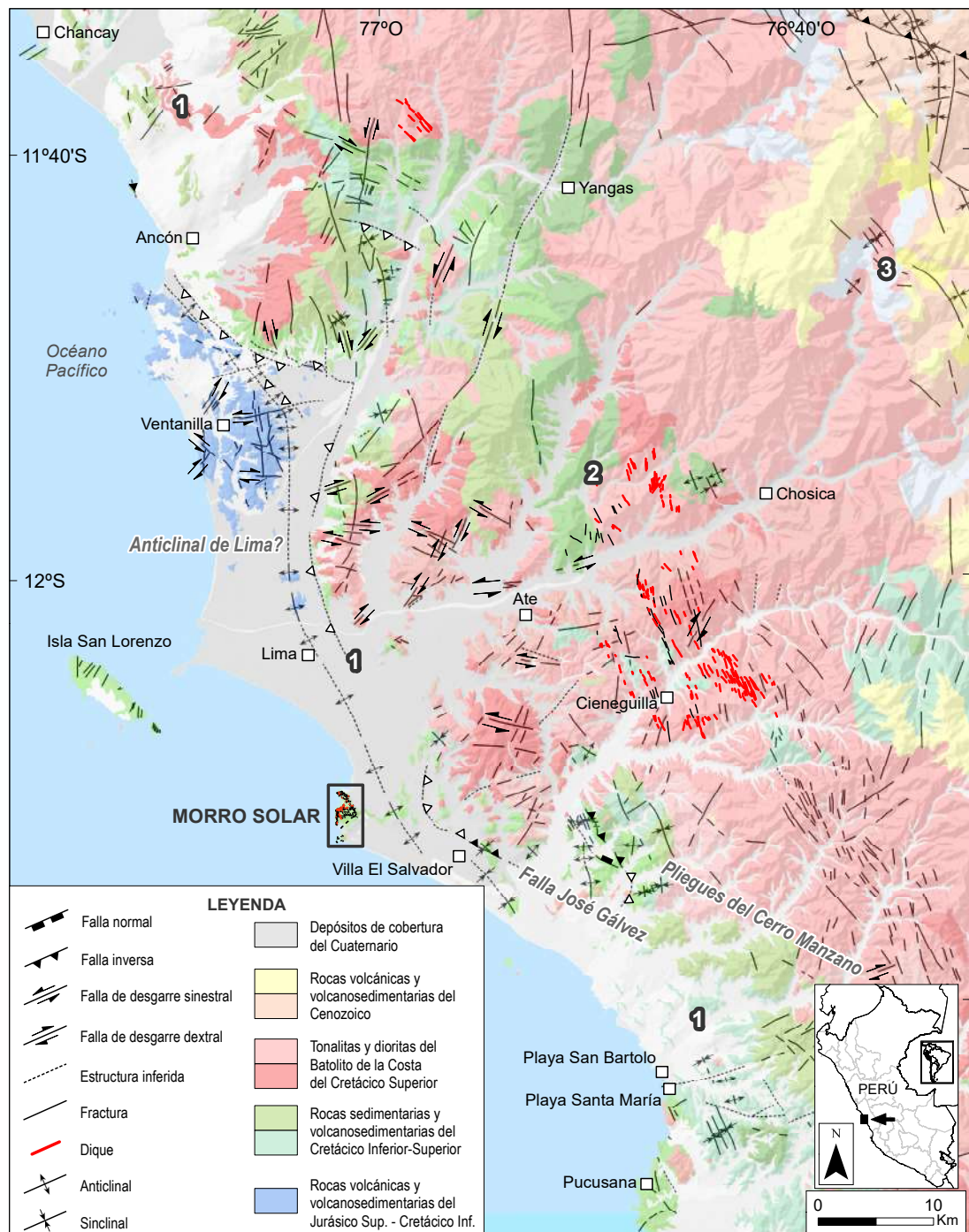
Figura 23. Mapa geológico regional de Lima entre las latitudes 11°30'S y 12°30'S (1: Antearco, 2: Vertiente Pacífica de la Cordillera Occidental Andina, 3: Cordillera Occidental). Compilado de Pardo (1961), Caldas (1980), Palacios et al. (1981), Figueroa (1988), Palacios (1992), Palacios et al. (1992) y Caldas y Palacios (1998).
