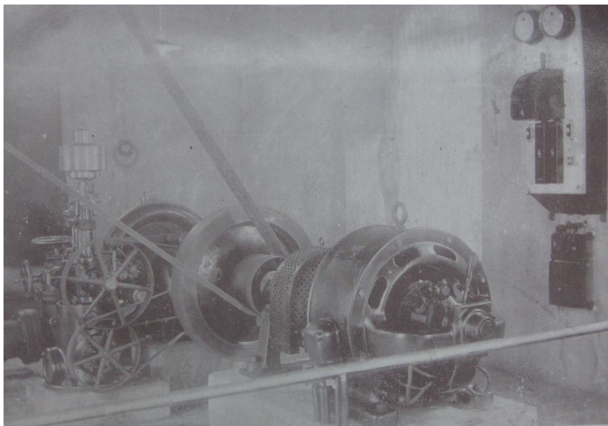
Figura 31. Turbinas de la oficina hidroeléctrica en los interiores de la “casa de agua”. Fuente: Gallese (1913).
