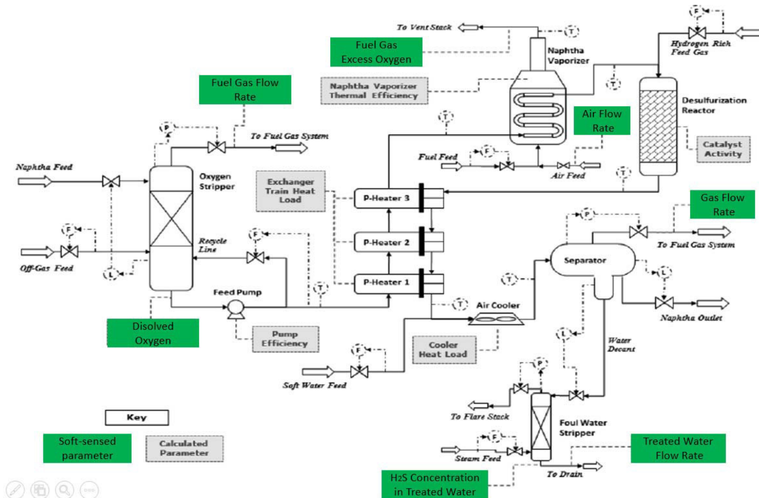
Figura 8 Ejemplo un simulador de procesos avanzado en tiempo real que integra la aplicación de los sensores virtuales (soft sensor) y también calcula parámetros de rendimiento/eficiencia para el proceso de endulzamiento de nafta. Fuente: Chowdhary A. R., 2014.
