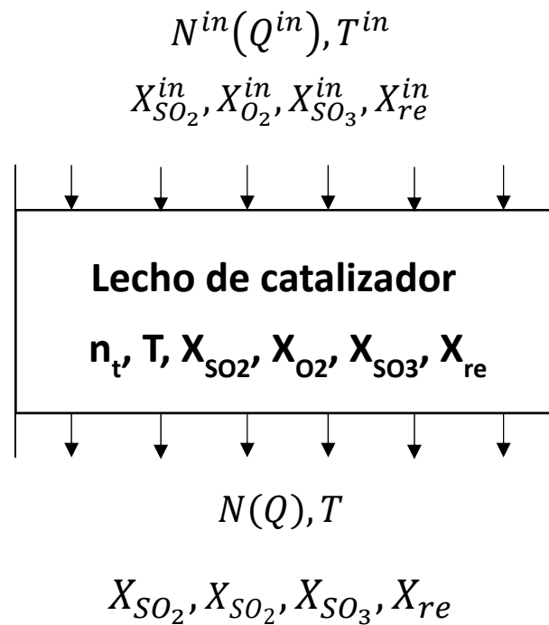
Figura A1.1 Esquema de variables en el lecho del convertidor
